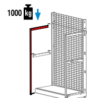
Stützrohr für hohe Lasten
